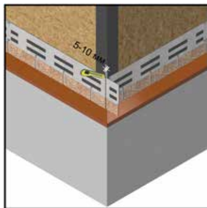
Рис. 14 Подрезка фасадной плитки к углам.
